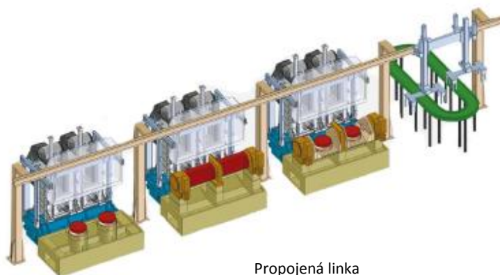
Propojená linka s automatickým zakladačem
