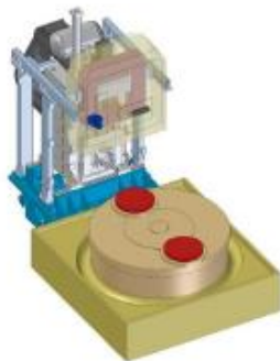
Rotační stůl B osa s výměnou palet
