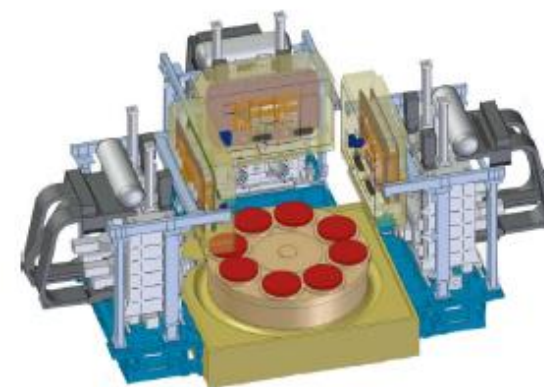
Rotační linka včetně B osy
