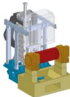
Sklopný příčník jako rotační horizontální osa A
