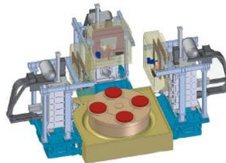
Rotační linka včetně B osy
